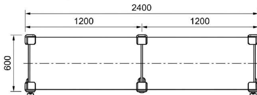
MẶT BẮNG (Ghép 1 khung)
