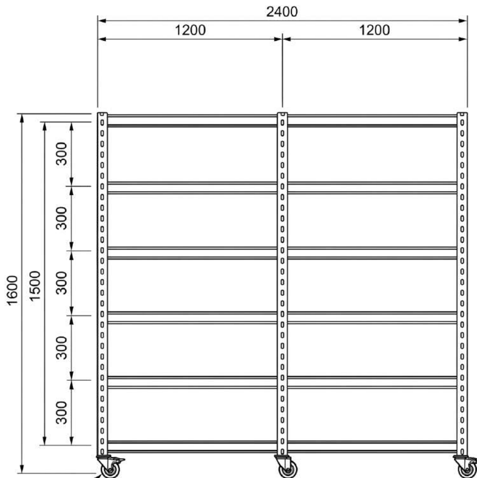
MẶT TRƯỚC (Ghép 1 khung, 3 chân)
